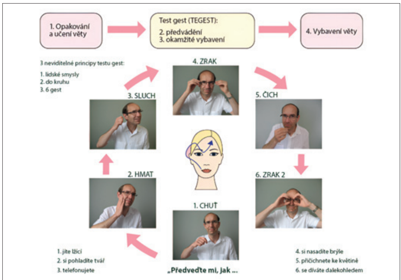
Obr. 1. Schéma testu ALBA.
