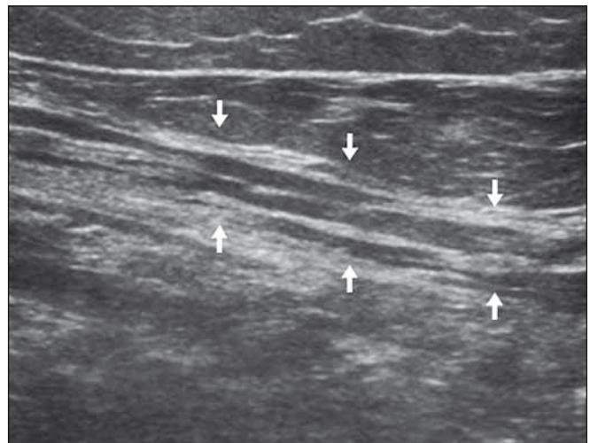
Obr. 8. Obraz nervu při CIDP (chronická zánětlivá demyelinizační polyneuropatie).
